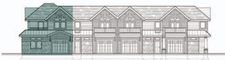
2 EXTERIOR ELEVATION - BLDG. 1 A-200 1/8"=1'-0"
